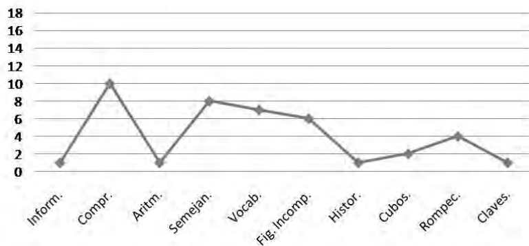
Gráfico 2. Perfil WISC-R.
